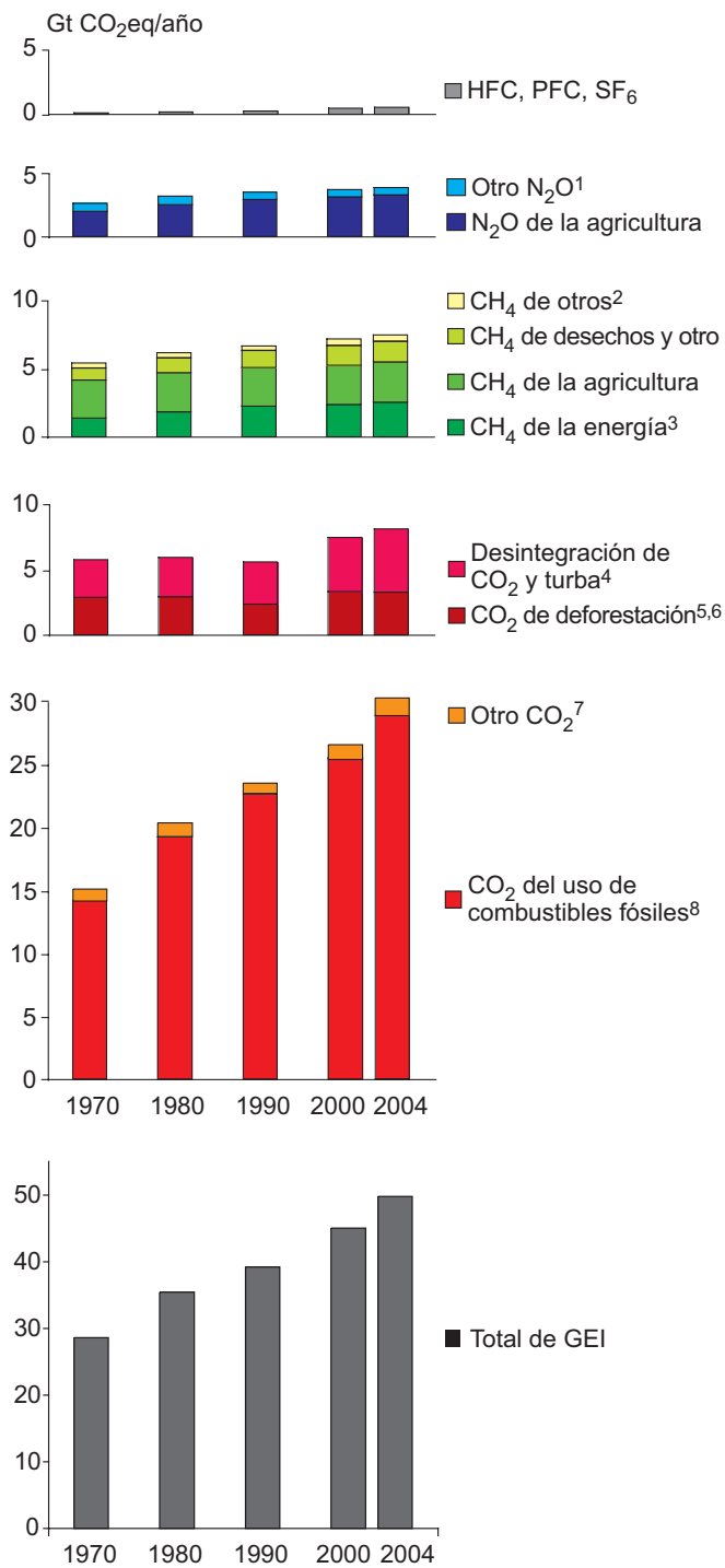
Gráfico RT.1a: Emisiones mundiales de gases de efecto invernadero antropogénicos, 1970-2004. Se utilizaron potenciales de calentamiento mundial (PCM) de 100 años del IPCC 1996 (SIE) para convertir emisiones en CO 2 -eq. (Véanse las directrices de la CMCC para la presentación de informes). Los gases son aquellos incluidos en las directrices de la CMCC para la presentación de informes. La incertidumbre en el gráfico es mayor para el CH 4 y N 2 O (del orden del 30-50%) y aún mayor para el CO 2 procedente de agricultura y silvicultura. [Gráfico 1.1a]
